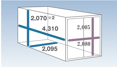
D ワイドキャブ/ロングボデー
