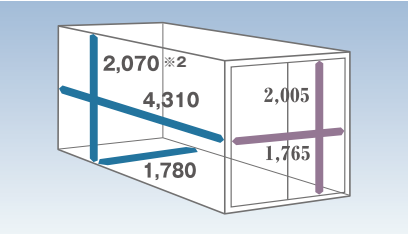
C 標準キャブ/ロングボデー
