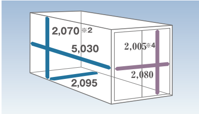
E ワイドキャブ/超ロングボデー
