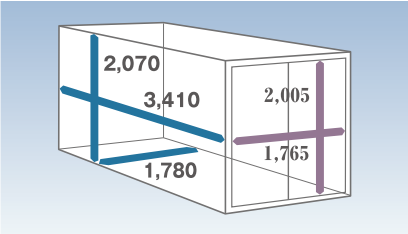
B 標準キャブ/セミロングボデー
