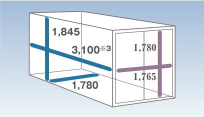
A 標準キャブ/標準ボデー
